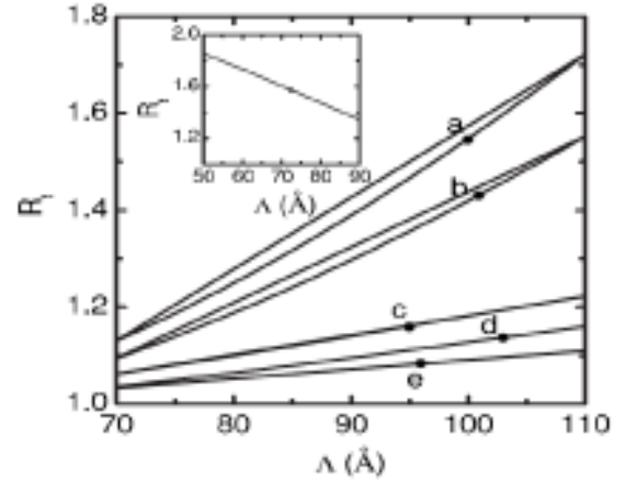
Hình 4.3 tỷ số thời gian sống vận chuyển phụ thuộc vào độ dài tương quan \Lambda trong mô hình trong giếng lượng tử AlAs/ GaAs/ AlAs.
