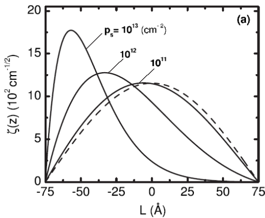
Hình 2.5(a) Đồ thị của hàm sóng với L=150\text{Å} , p_s=10^{11}, 10^{12}, 10^{13}\text{cm}^{-2}
