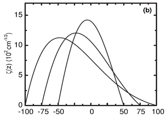
Hình 2.5(b) Đồ thị của hàm sóng với p_s = 5.10^{11}\text{cm}^{-2} , L = 100, 150, 300\text{Å}
