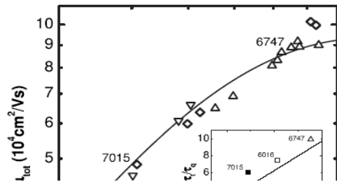
Hình 2.9 Độ linh động trong giếng lượng tử Si 0.3 Ge 0.7 /Ge/Si 0.3 Ge 0.7 pha tạp một phía.
