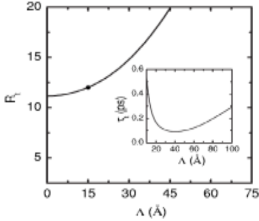
Hình 4.2 Tỷ số thời gian sống vận chuyển phụ thuộc vào độ dài tương quan \Lambda trong giếng lượng tử GaSb/ InAs/ GaSb.
