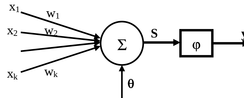
Hình 1.4. Mô hình một nơron nhân tạo
