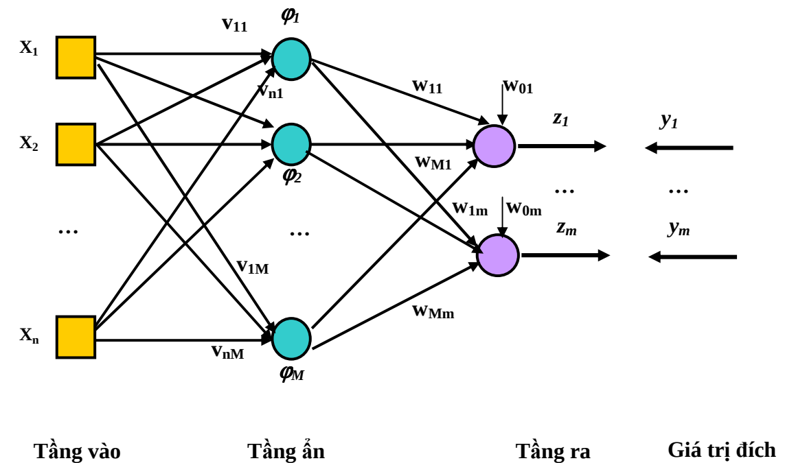
Hình 2.5 Mô tả kiến trúc mạng nơron RBF
