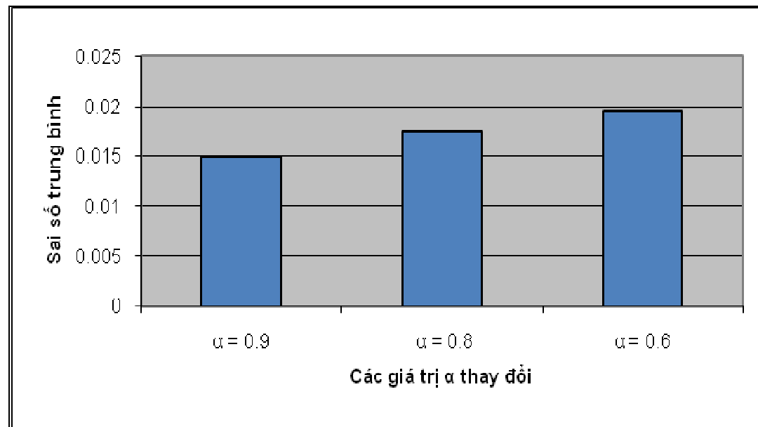
Hình 3.6 Đồ thị kiểm tra sai số khi \alpha thay đổi
