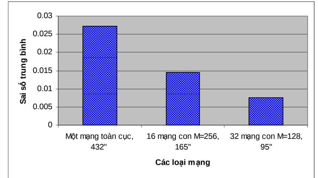
Hình 5.7: Đồ thị so sánh tính tổng quát hoá với hàm 2 biến có 4086 mốc nội suy tại 10 điểm xa tâm.
