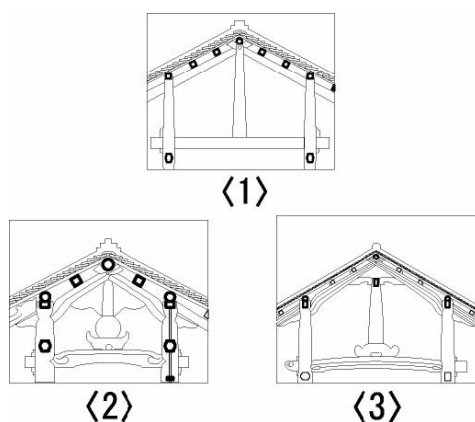
Hình 5: Cấu tạo chi tiết liên kết phần nóc mái giữa trụ , kèo và đòn dông
