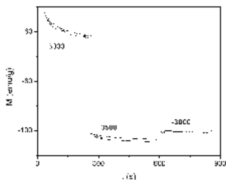
Hình 9. Sự suy giảm từ độ theo thời gian dưới tác dụng của từ trường ngược -3 kOe và -3,5 kOe. Thời gian thay đổi từ trường là 350 s.
