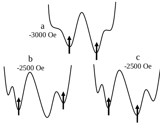
Hình 8. Giảm đồ năng lượng của hệ nano tổ hợp phụ thuộc vào từ trường ngoài: (a) -3000 Oe; (b, c) -2500 Oe.
