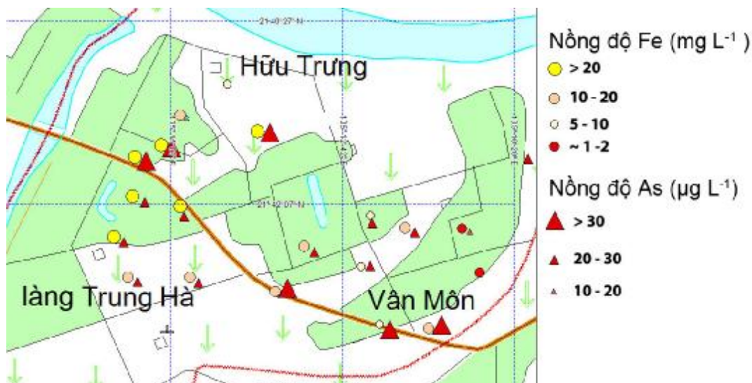
Hình 4. Biểu đồ biểu diễn hàm lượng As và Fe trong các mẫu nước nghiên cứu.
