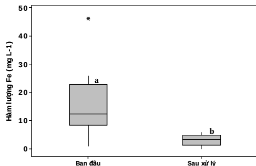
Hình 3. Hàm lượng Fe và As trước và sau xử lý của các hộ gia đình khu vực nghiên cứu.
