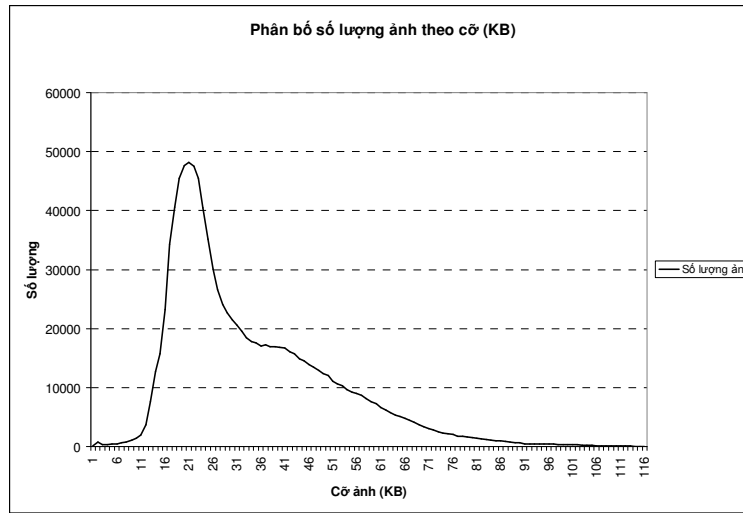
Hình 4. Phân bố số lượng ảnh tile theo cỡ.
