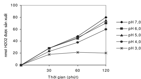
Hình 1. Khả năng sản xuất \text{H}_2\text{O}_2 của chủng S. sobrinus ATCC 6715 ở các pH khác nhau.
