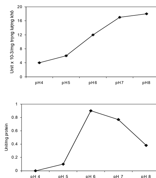
Hình 4. Hoạt độ NADH oxidase của tế bào thẩm (A) và của dịch chiết (B) tế bào S. sobrinus .
