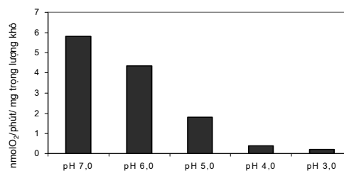
Hình 2. Khả năng hô hấp của S. sobrinus 6715 tại các pH khác nhau.
