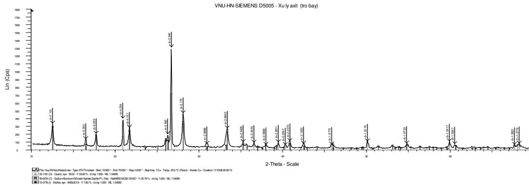
Hình 2. Phổ nhiễu xạ tia X tro than bay sau xử lý.
