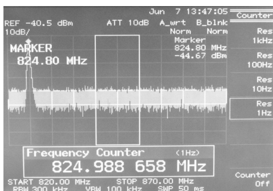
Hình 9. Tần số dao động trên máy phân tích phổ R3131A.
