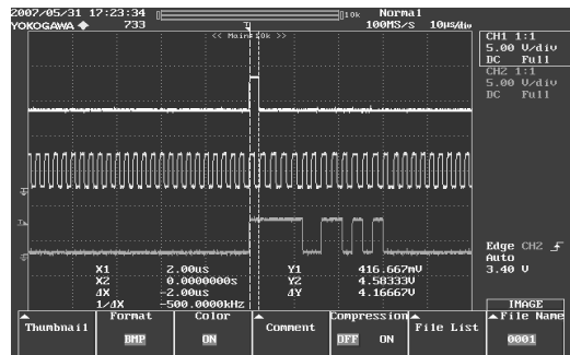
Hình 6. Mã Barker N = 13.
