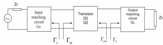
Hình 4. Mô hình khối khuếch đại công suất.
