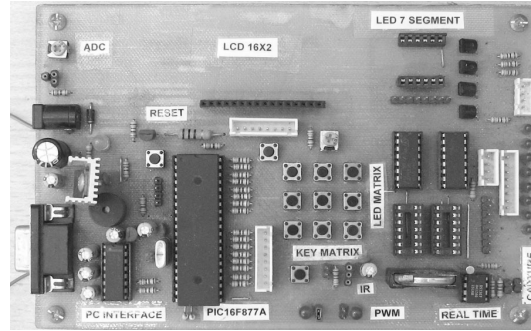
Hình 5. Kít phát triển PIC16F877A.
