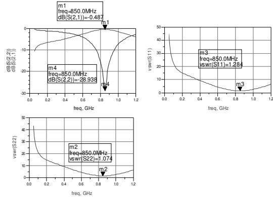
Hình 12. Các tham số S mô phỏng tại 850MHz.
