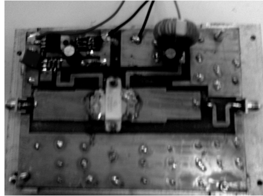
Hình 13. Khối khuếch đại công suất cao tần dùng mạch dài.
