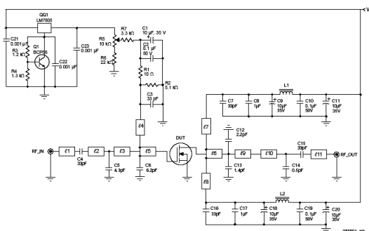
Hình 10. Sơ đồ nguyên lý mạch khuếch đại công suất cao tần.
