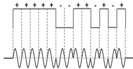
Hình 2. Mã Barker 13 bit và tín hiệu BPSK tương ứng.
