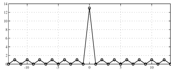
Hình 3. Hàm tự tương quan của mã Barker 13 bit.
