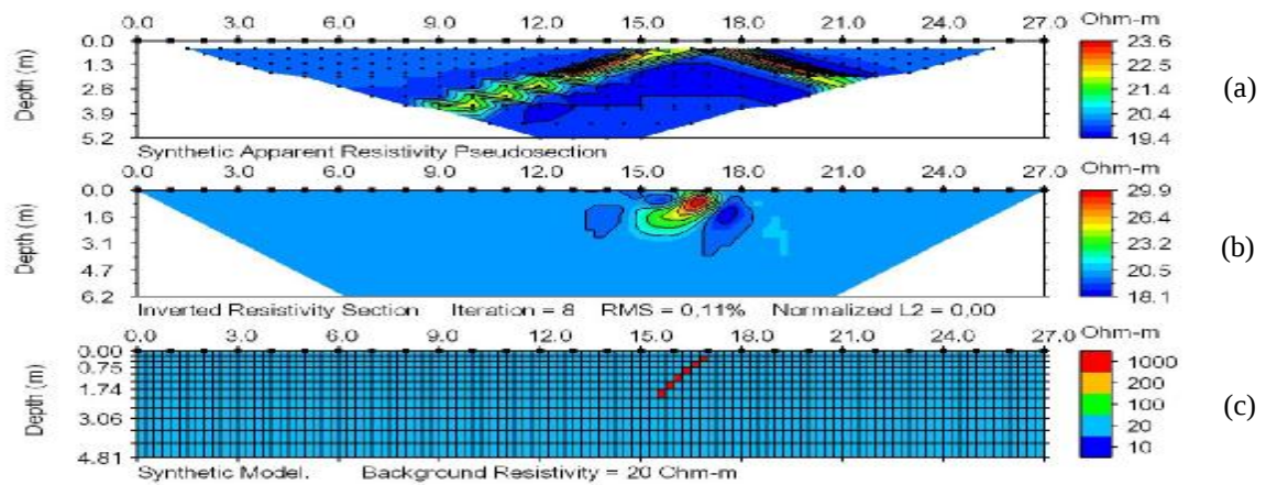
Hình 2. Tính lý thuyết khe nứt nghiêng 45^\circ với hệ cực dipole-dipole.
