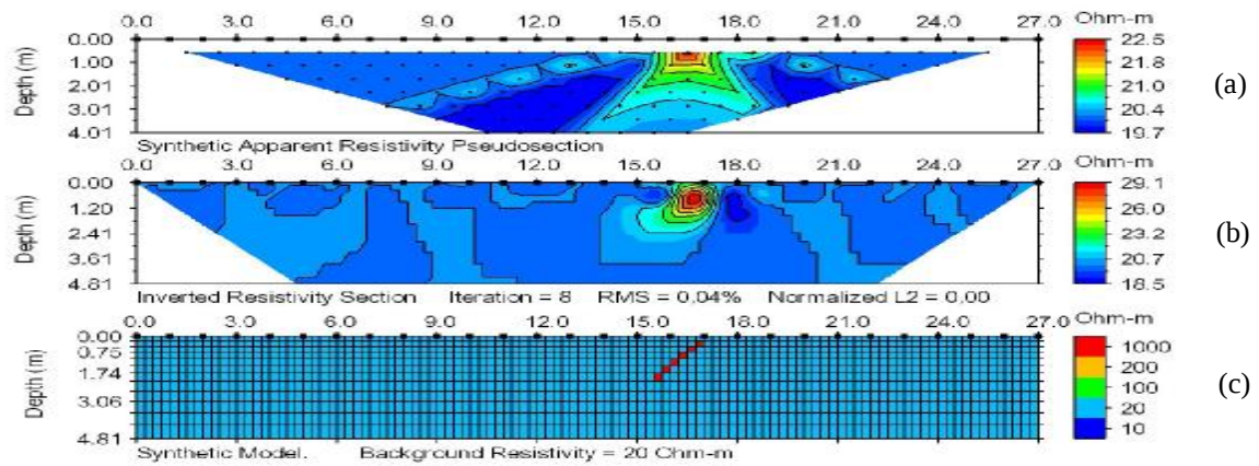
Hình 3. Tính lý thuyết khe nứt nghiêng 45^\circ với hệ cực Wenner.
