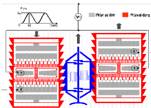
Hình 4. Môđun đi thẳng.
