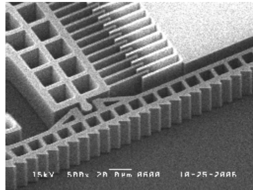
Hình 8. Cơ cấu kích hoạt kiểu răng lược và thanh răng cóc.
