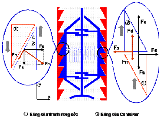
Hình 6. Các lực tác động trên hệ thống.
